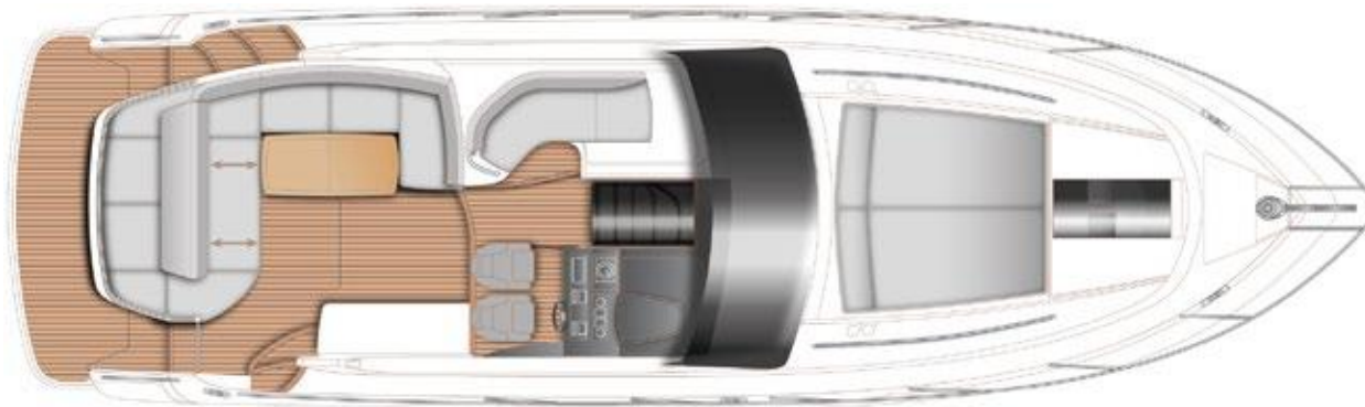
ГЛАВНАЯ ПАЛУБА (ОПЦИЯ)
