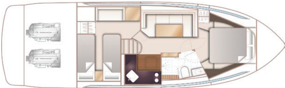
НИЖНЯЯ ПАЛУБА
